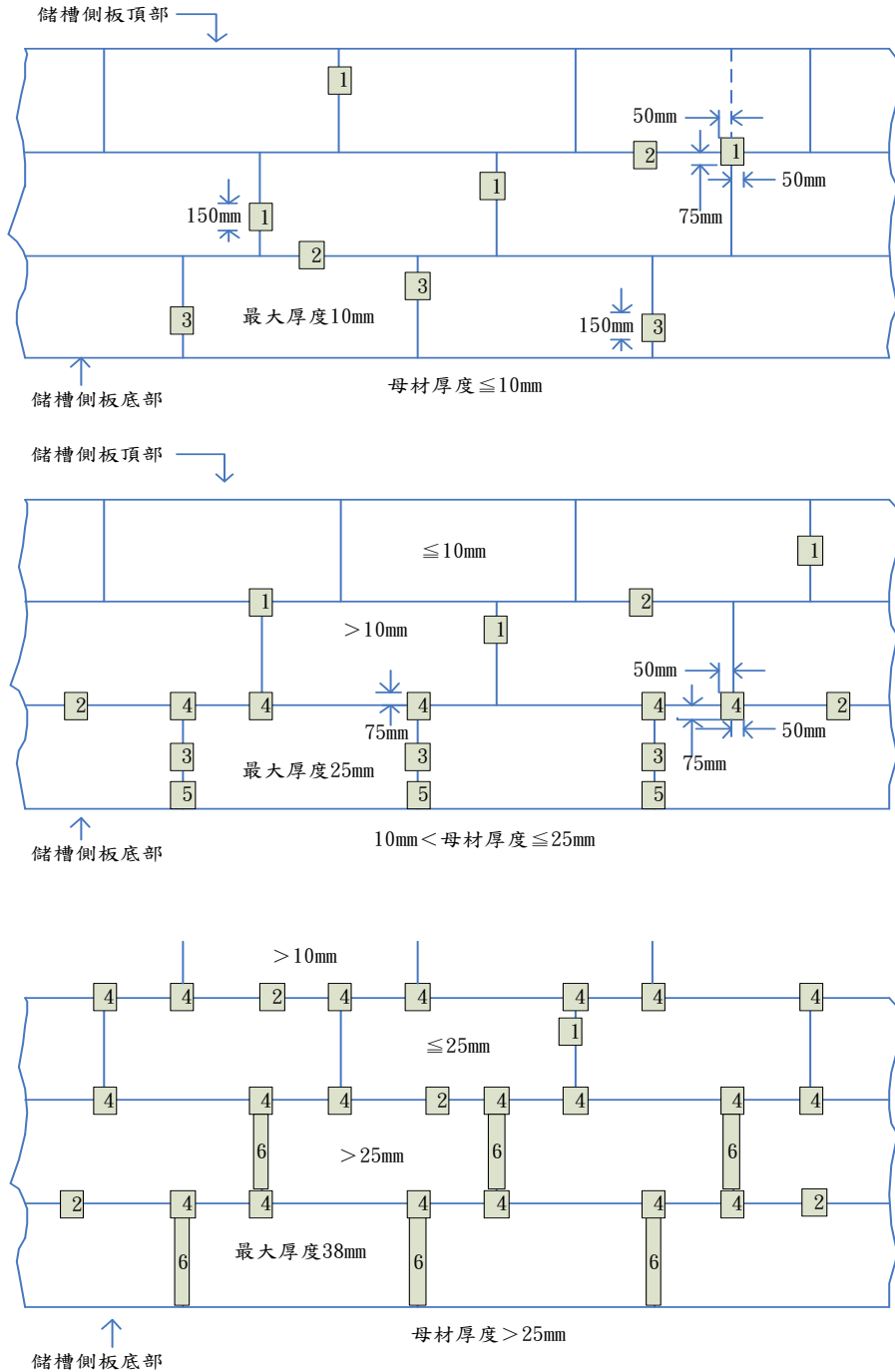
放射線透過試驗攝影位置圖示 (圖中方格內編號之說明如備註)
