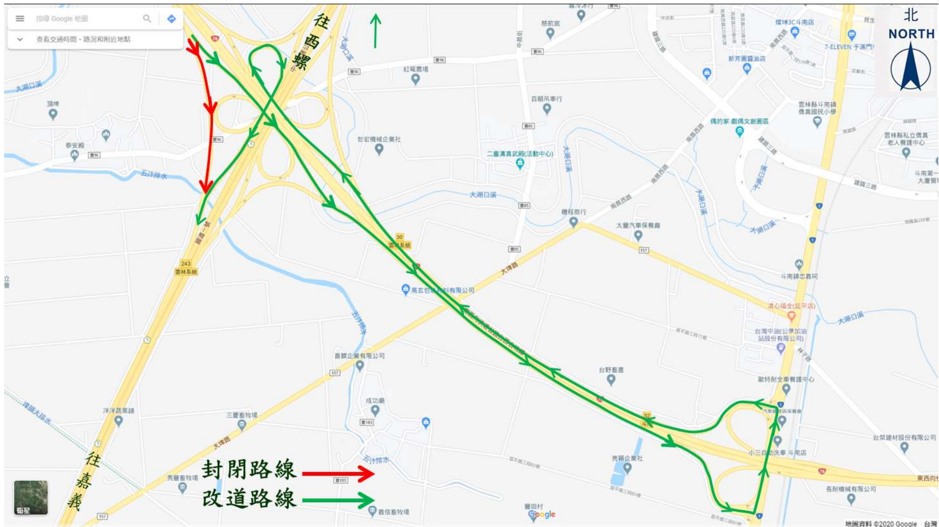
(圖三)台 78 線東行往國道 1 號雲林系統交流道南下入口匝道改道路線圖
