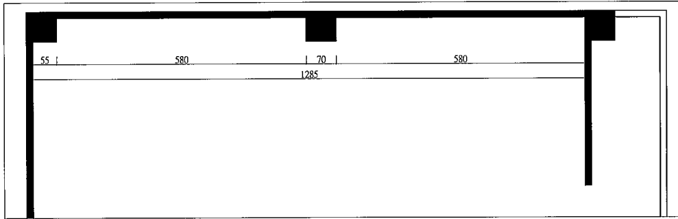
02 一樓第一展示室B向立面圖 S:1/60
