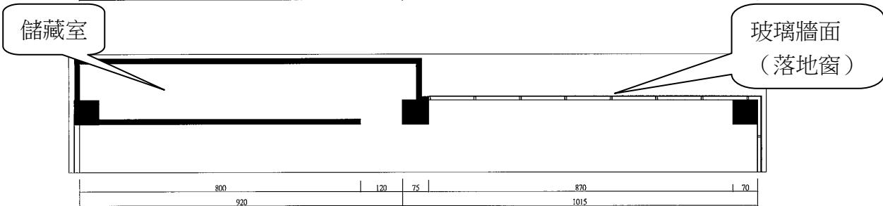
03 一樓第一展示室C向立面圖 S:1/60
