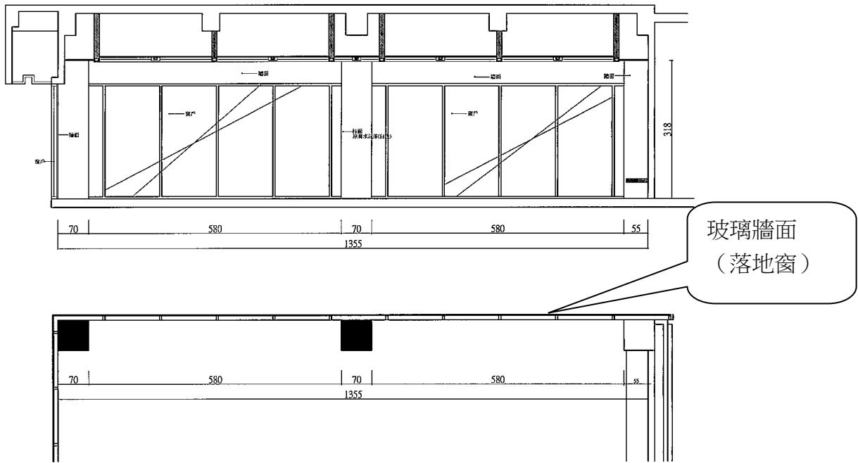
04 一樓第一展示室D向剖面圖 S:1/60
