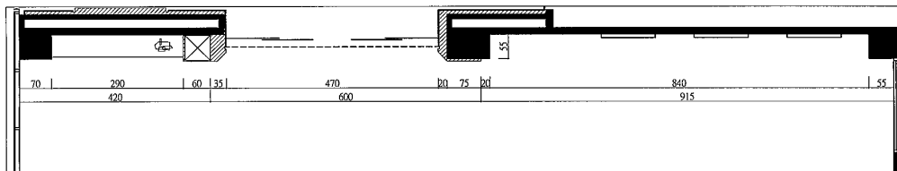
01 一樓第一展示室A向立面圖 S:1/60
