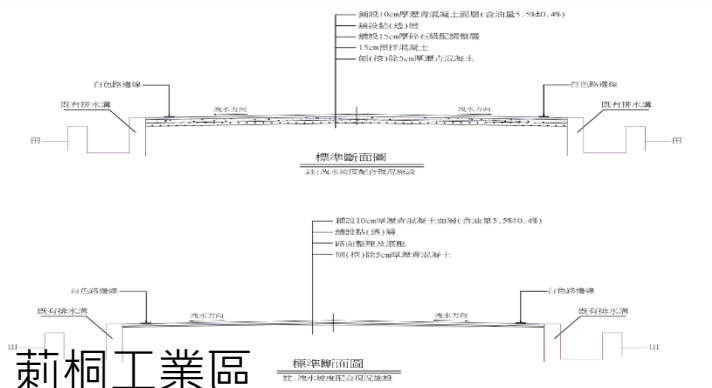
道路工程標準斷面圖
