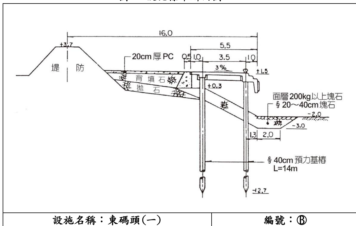
圖5 設施標準斷面圖 2
