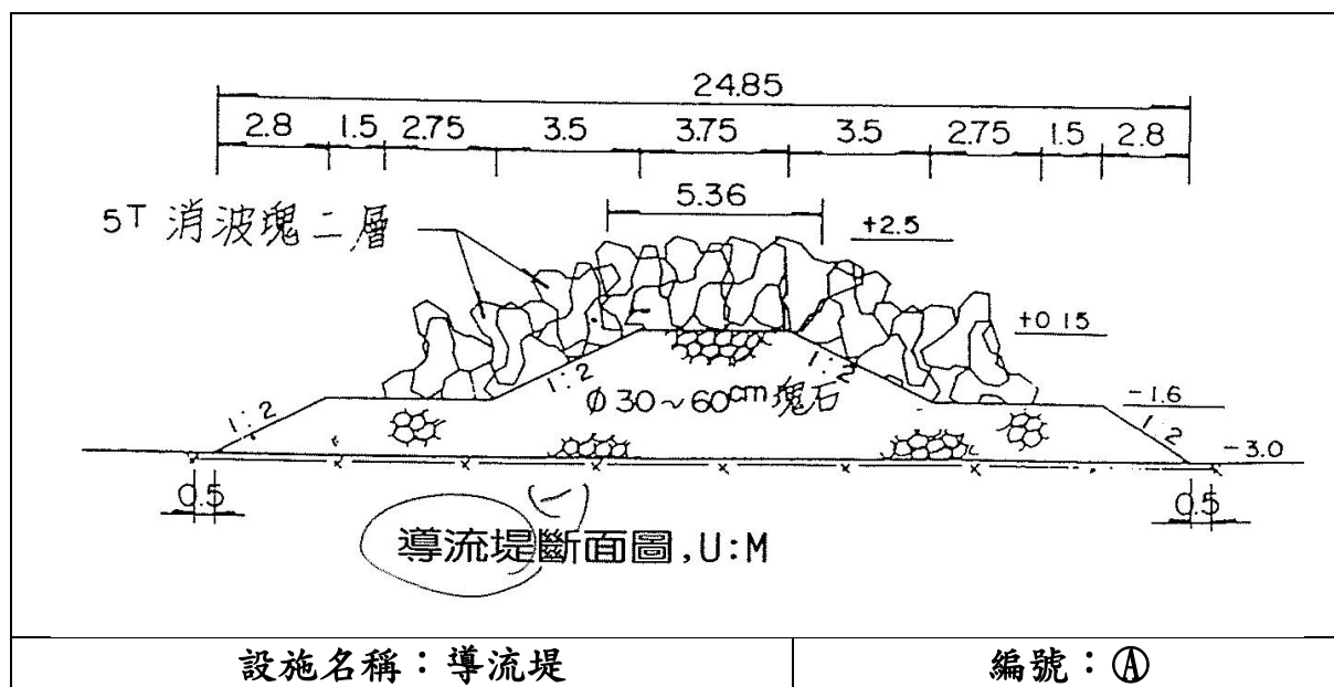
圖4 設施標準斷面圖 1
