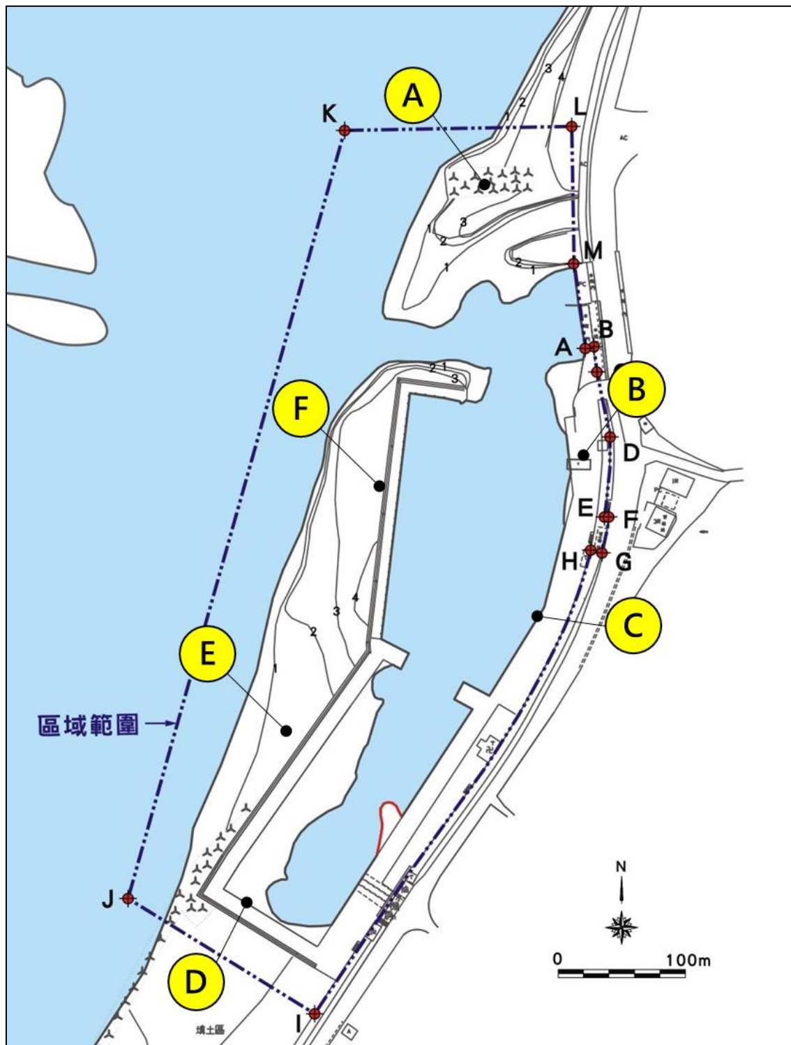
圖3 塭豐漁港設施斷面位置圖
