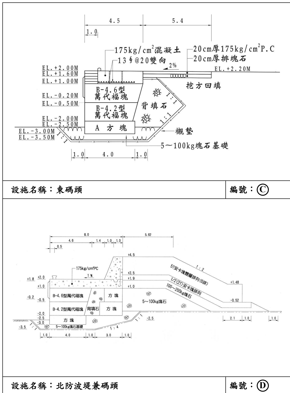
圖 6 設施標準斷面圖(續一)
