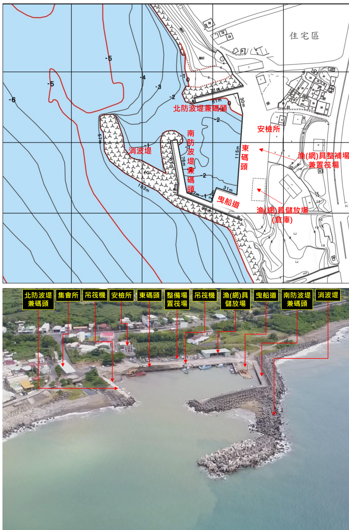
圖4 楓港漁港設施位置示意圖
