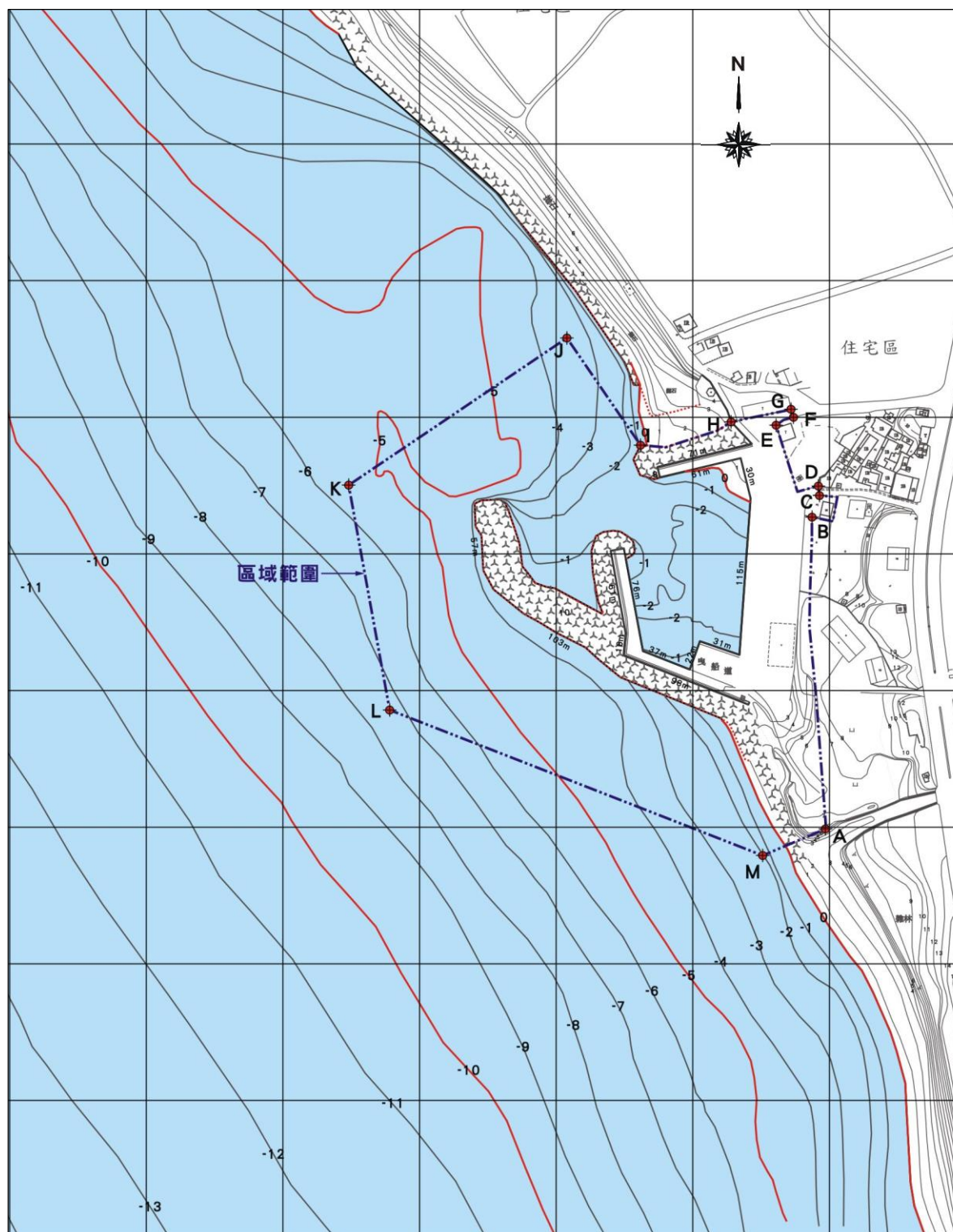
圖1 楓港漁港區域平面圖
