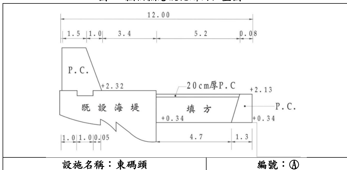
圖5 設施標準斷面圖
