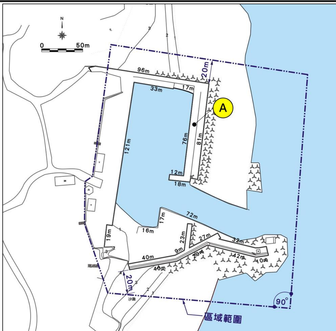
圖4 漁福漁港設施斷面位置圖
