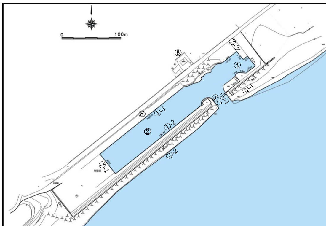
圖2 中山漁港設施位置示意圖
