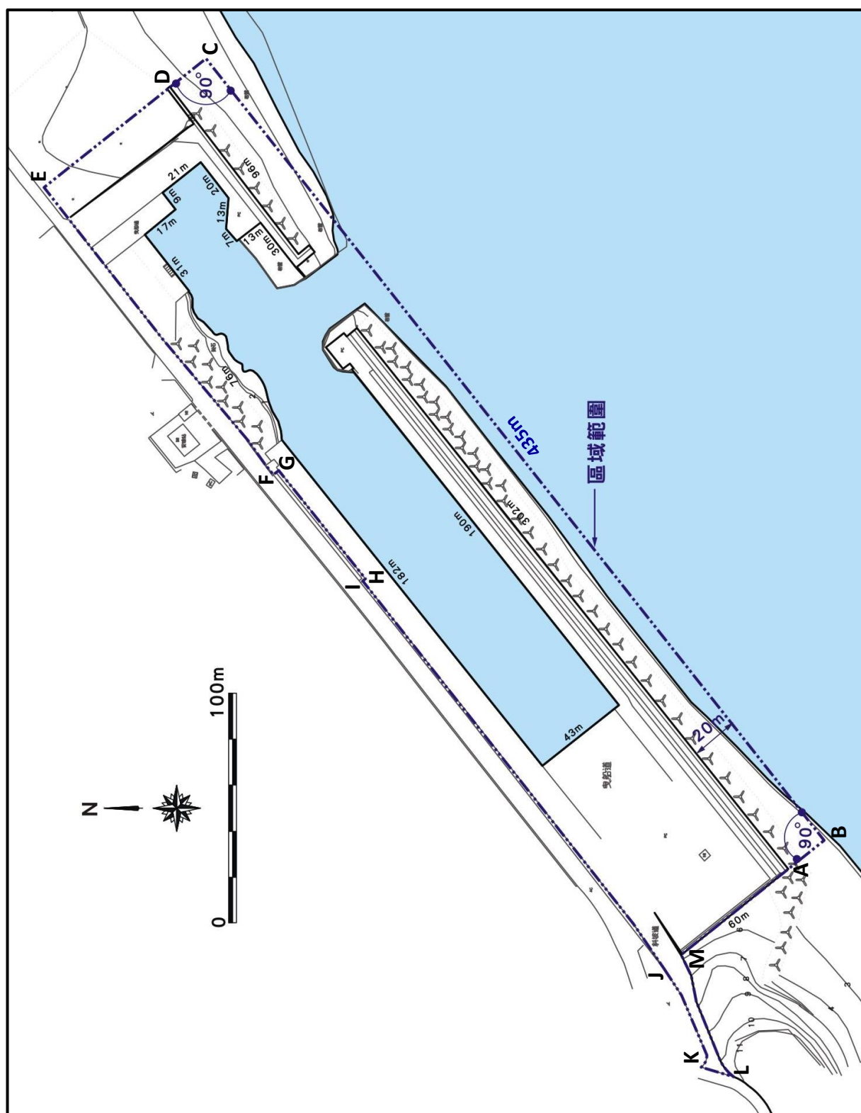
圖1 中山漁港區域範圍平面圖
