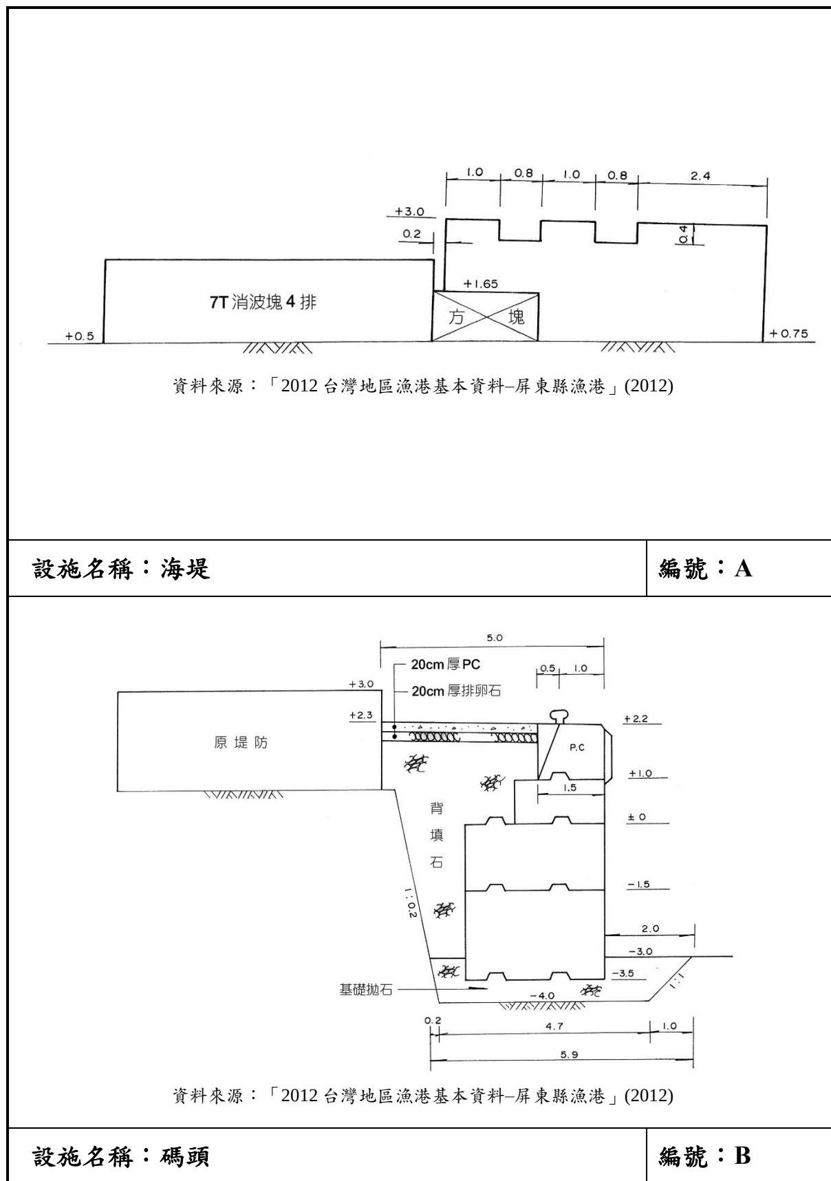
圖4 旭海漁港設施標準斷面圖
