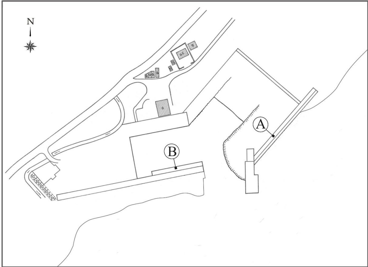
圖3 旭海漁港設施斷面位置圖
