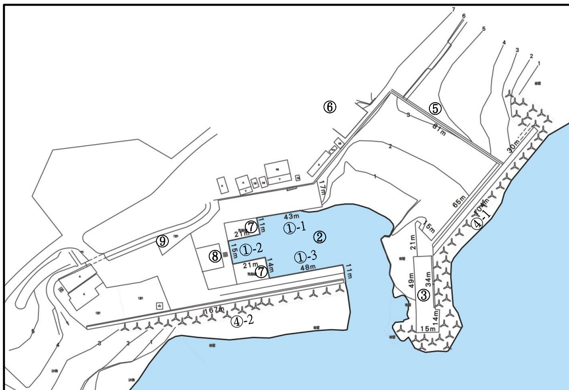
圖2 旭海漁港設施位置示意圖
