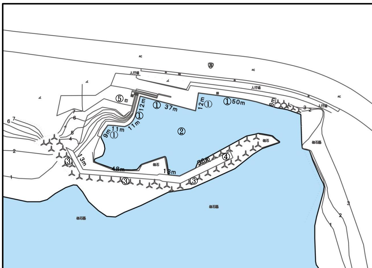
圖3 潭仔漁港設施位置示意圖
