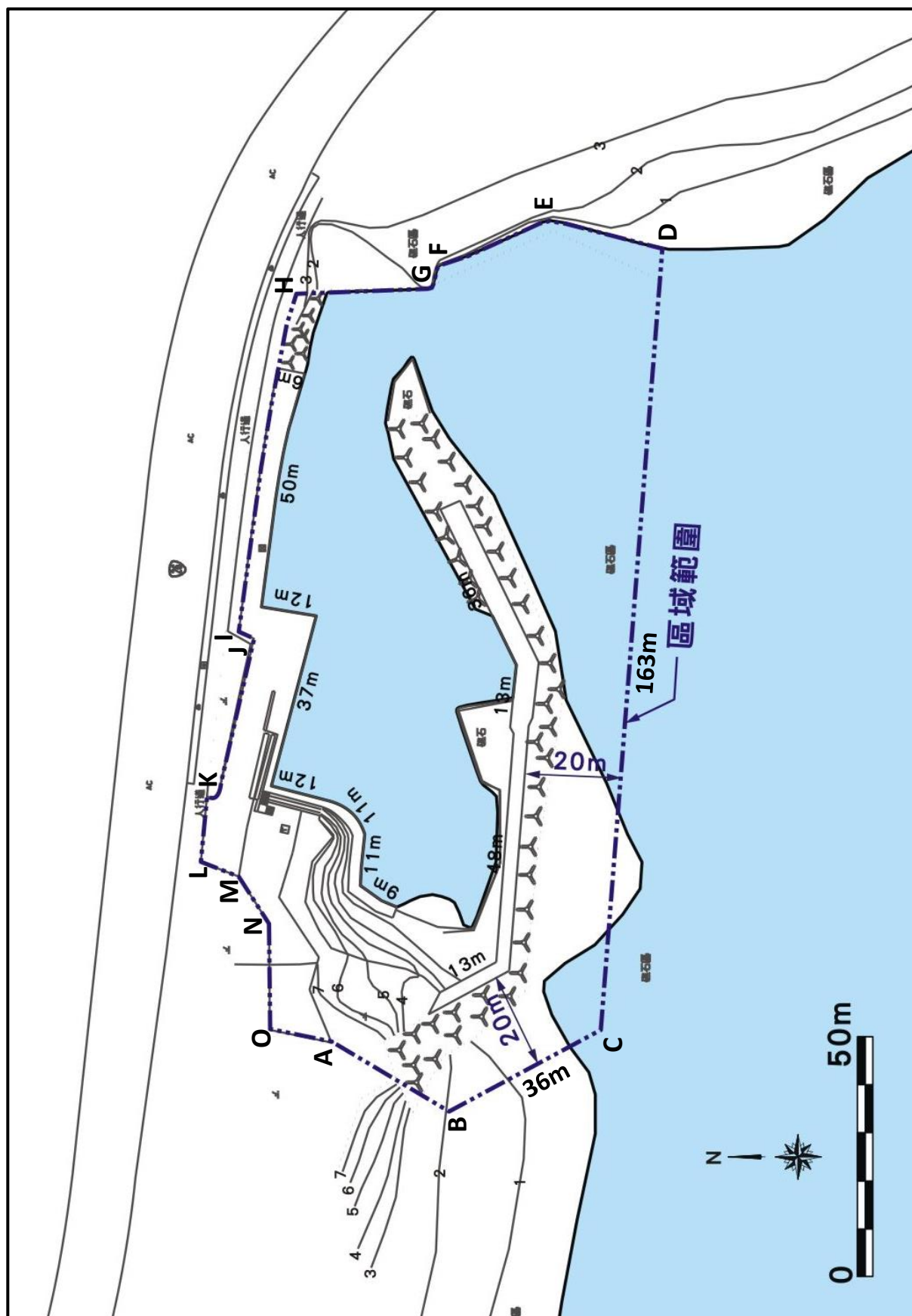
圖1 潭仔漁港區域範圍平面圖
