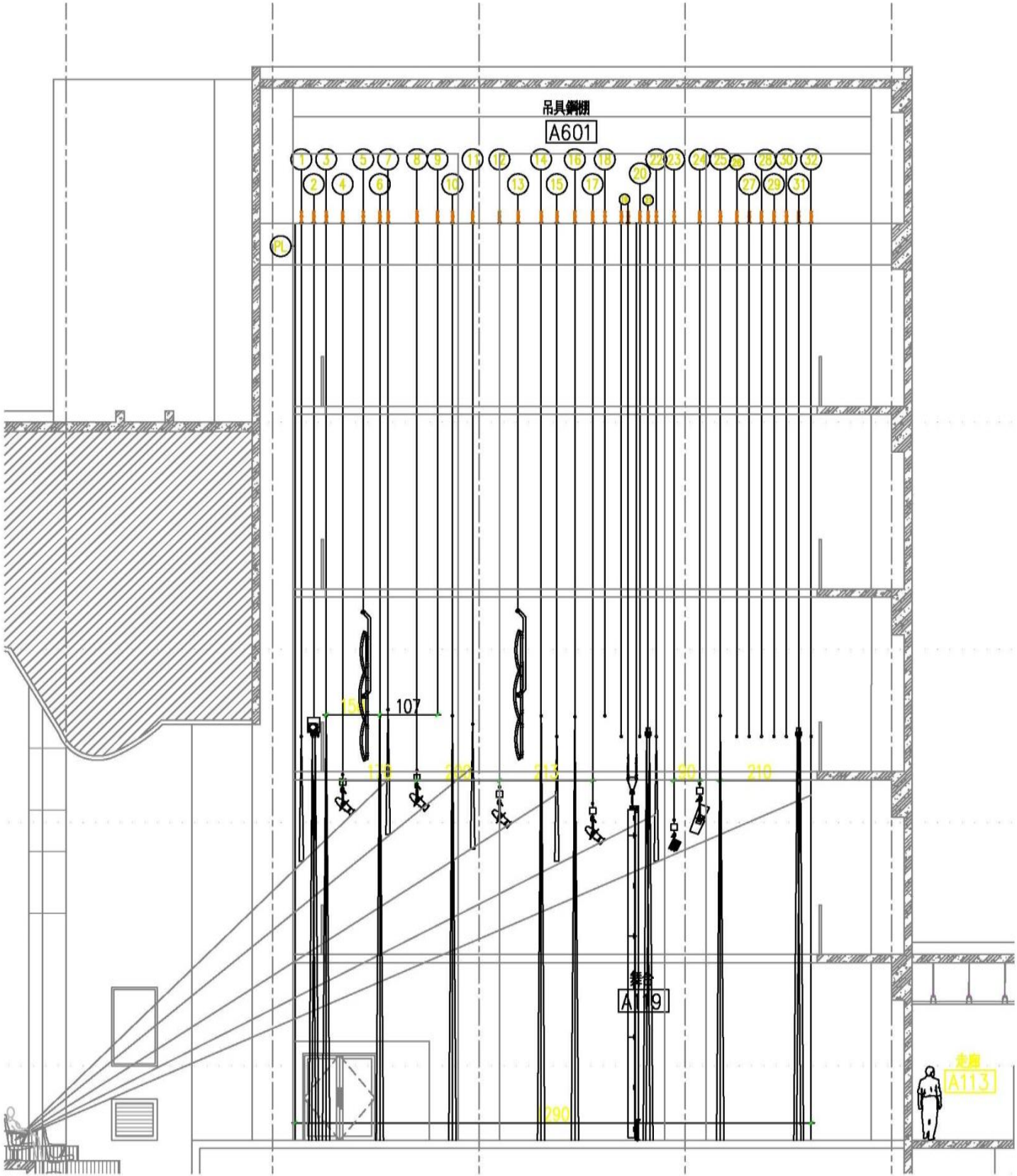
舞台懸吊立面配置圖
